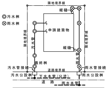
□ 排水接続 (分流・雨水は雨水本管接続)
