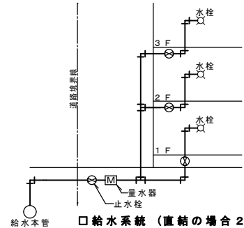
□ 給水系統 (直結の場合2)
