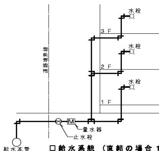
□ 給水系統 (直結の場合1)
