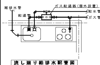
流し廻り給排水配管図
