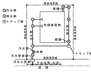
□ 排水接続 (合流・雨水共下水本管放流)
