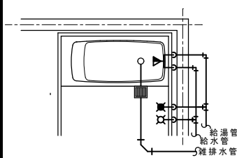
浴室廻り給排水配管図
