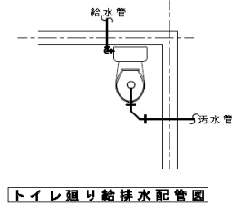
トイレ廻り給排水配管図
