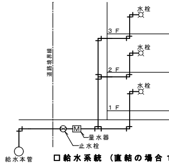
□ 給水系統 (直結の場合1)
