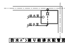
防水ハシ廻り給排水配管図
