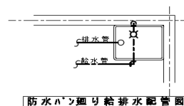
防水パッキン廻り給排水配管図
