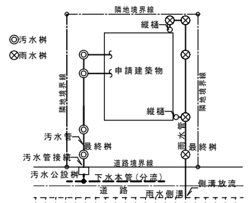
□ 排水接続 (分流・雨水は側溝に放流)
