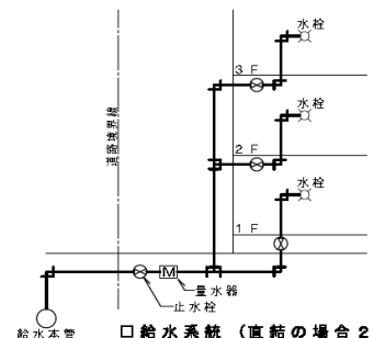
□ 給水系統 (直結の場合2)
