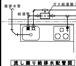
流し廻り給排水配管図
