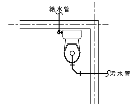
トイレ廻り給排水配管図
