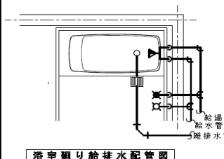
浴室廻り給排水配管図
