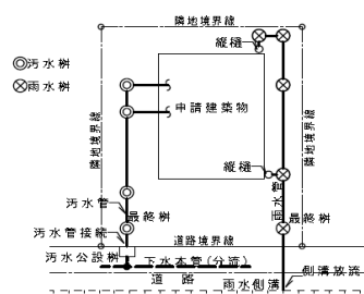
□ 排水接続 (分流・雨水は側溝に放流)
