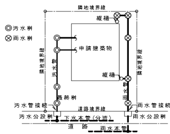
□ 排水接続 (分流・雨水は雨水本管接続)
