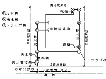
□ 排水接続 (合流・雨水共下水本管接続)
